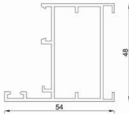
پروفیل فریم Frame Profile Code : 12312 weight : 0.8 kg/m
