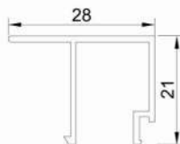
زهوار تک جداره rickety Code : 12353 weight : 0.22 kg/m
