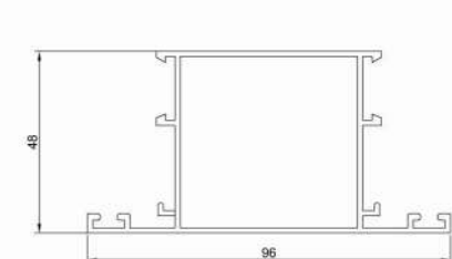
پروفیل سپری Tripetalous profile Code : 12441 weight : 1.14 kg/m
