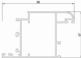
پروفیل لنگه Vent profile Code : 12431 weight : 1.3 kg/m
