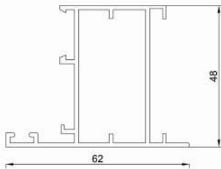
پروفیل فریم Frame Profile Code : 12311 weight : 0.84 kg/m
