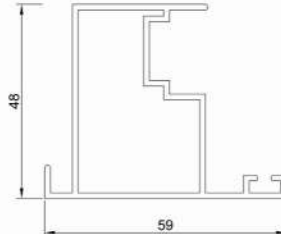
پروفیل وسط دو لنگه between the two vents Code : 12481 weight : 0.84 kg/m
